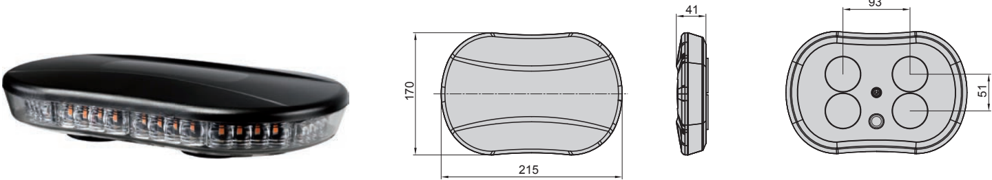
Fissaggio a 4 base magnetica - magnetic mount
