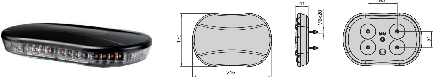
Fissaggio a 4 viti - 4 bolts fixing
