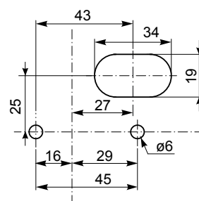
Foratura di applicazione Fixing hole
