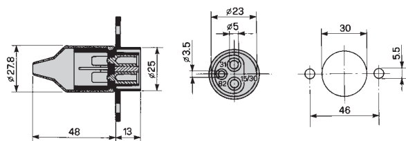
Uscite posteriori capicorda serie 6,35 e 4,8 Rear outputs terminals series 6,35 and 4,8
