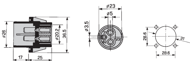
Uscite posteriori capicorda serie 6,35 e 4,8 Rear outputs terminals series 6,35 and 4,8
