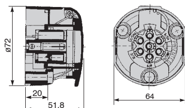
Uscite posteriori a vite Rear outputs screw
