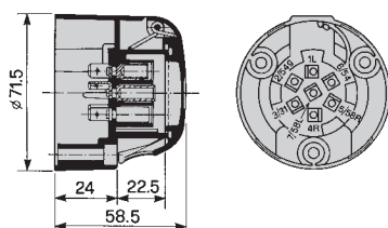
Uscite posteriori capicorda serie 6,35 Rear outputs terminals series 6,35
