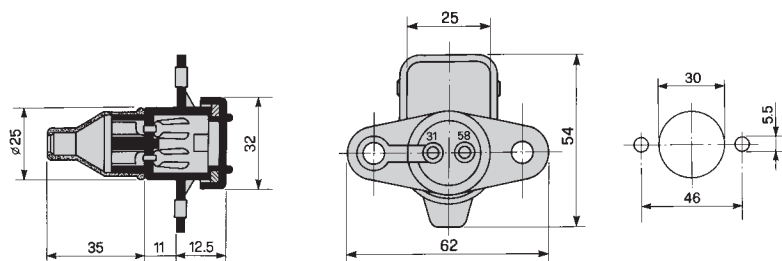
Uscite posteriori morsetti per capicorda a spina ø4 Rear outputs clamps for terminals plug ø4
