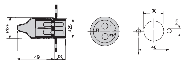
Uscite posteriori capicorda serie 6,35 Rear outputs terminals series 6,35
