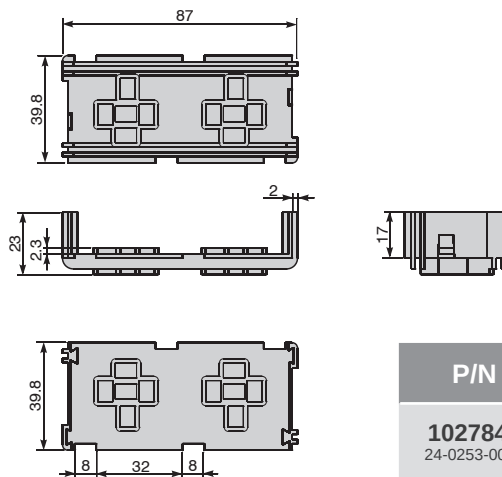
Supporto per Minirelè 30A Frame for 30A Mini Relays
