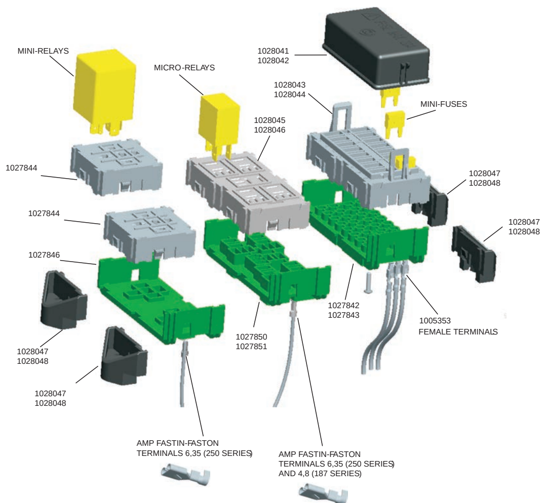
Esempio di Composizione Assembly Example
